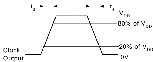
Figure 5. ER = (0.6 \times V_{DD})/t_3 , EF = (0.6 \times V_{DD})/t_4
