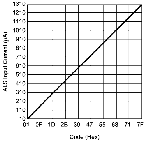
ALS Input Current vs Code V_{ALS} = 2V
