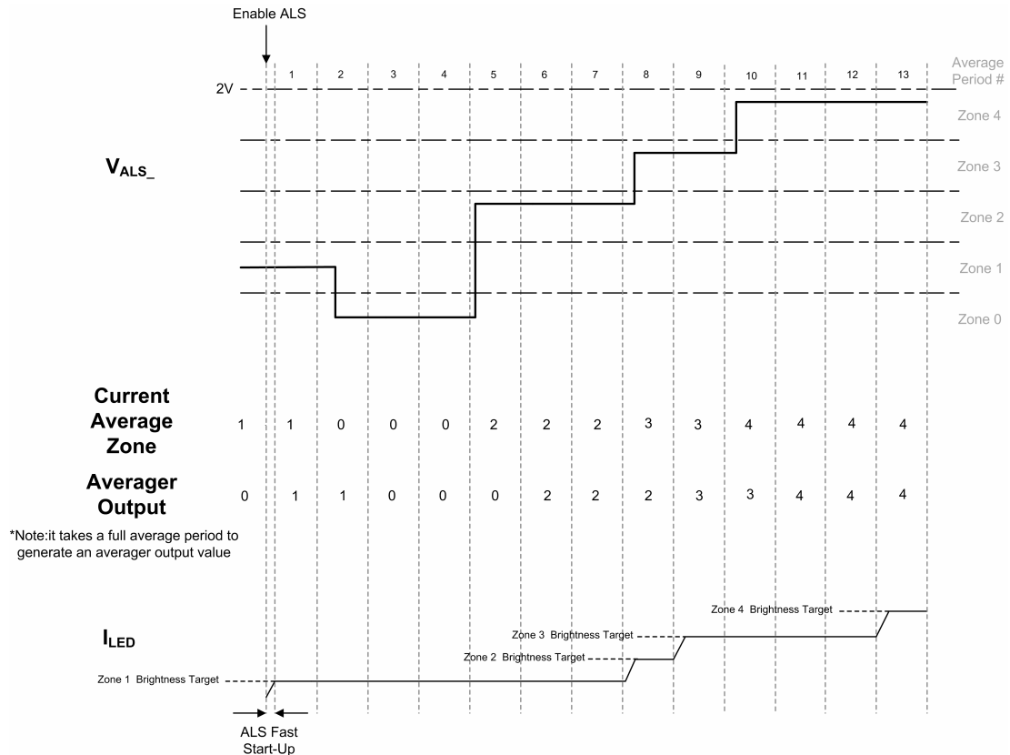
FIGURE 12. ALS Up-Only Control
