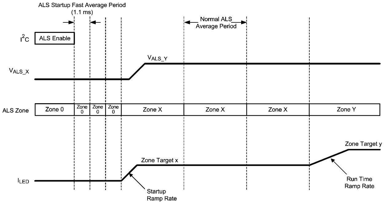
FIGURE 10. ALS Startup Sequence
