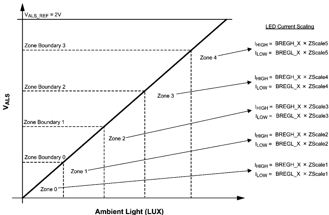
FIGURE 15. ALS Controlled Pattern Current Scaling
