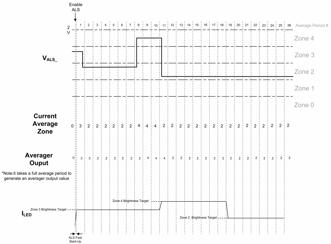
FIGURE 13. ALS Down-Delay Control
