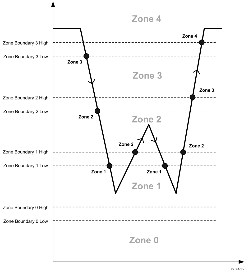
FIGURE 6. ALS Zone Boundary + Hysteresis
