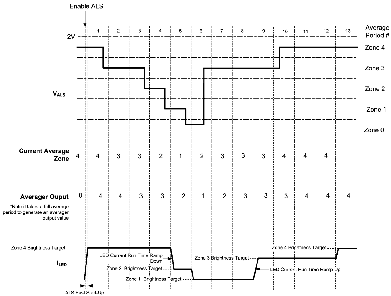
FIGURE 11. Direct ALS Control
