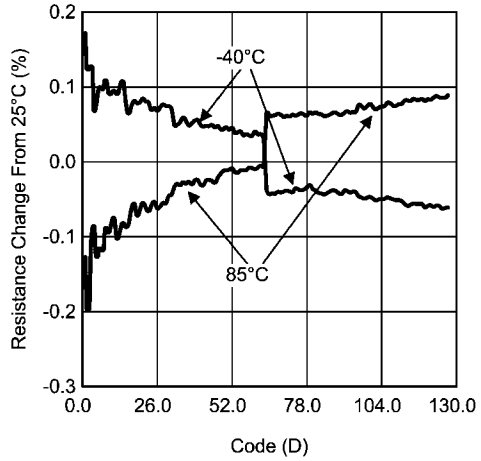
ALS Resistance vs Code (Temp)
