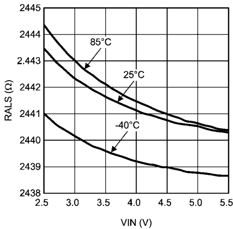
ALS Resistance vs VIN (Code 0x50)
